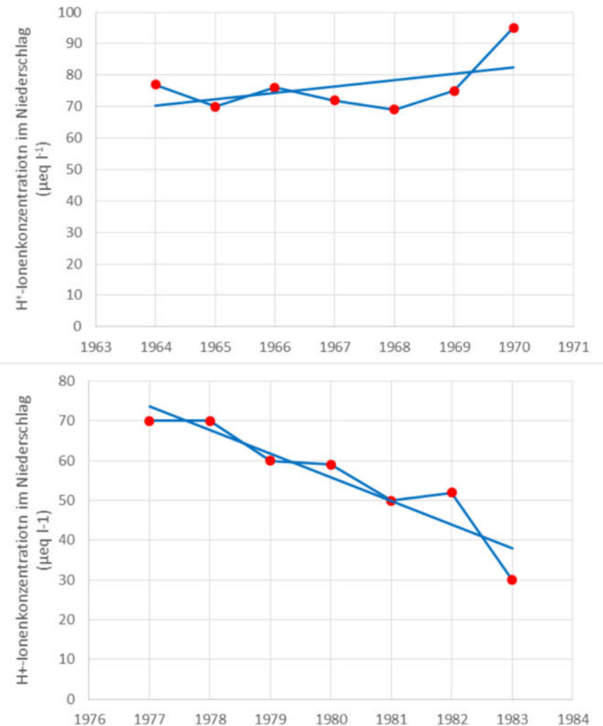
Säurekonzentration des Regens im Hubbart Brook Experimental Forest
